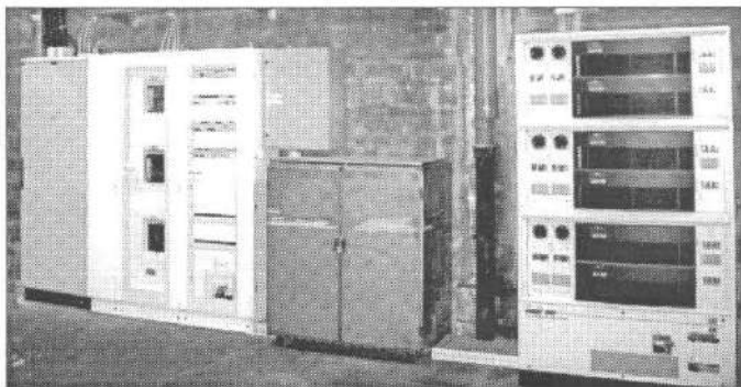
Primer uporabe modularnega – centraliziranega inverterja:
